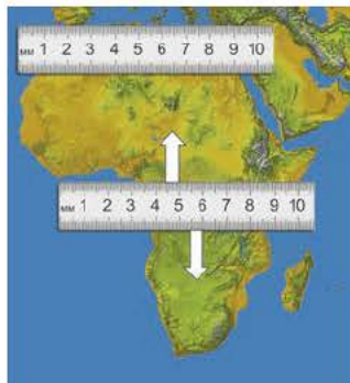
38-сурет. Материктің шеткі нүктесін табу
