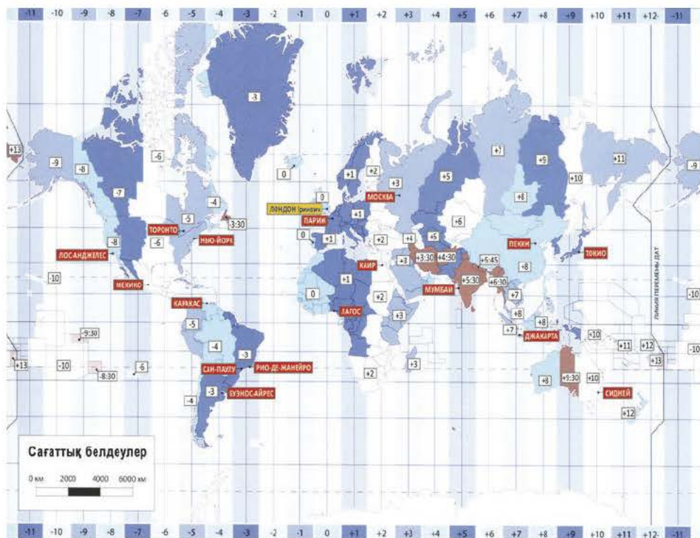
36-сурет. Дүниежүзіндегі сағаттық белдеулер картасы
