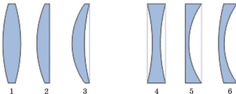
40.3-сурет. Линзаның түрлері: 1 — қосдөңес линза; 2 — жазық-дөңес линза; 3 — ойыс-дөңес линза; 4 — қосойыс линза; 5 — жазық-ойыс линза; 6 — дөңес-ойыс линза
