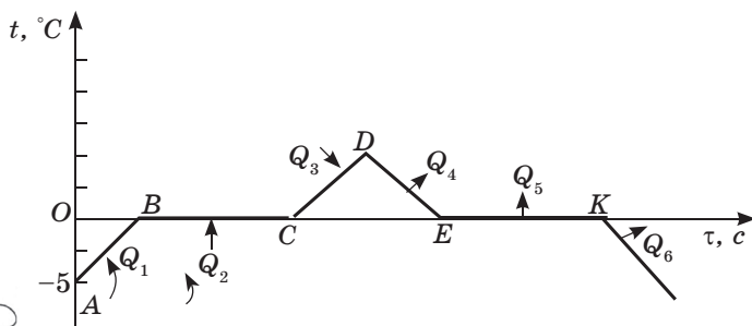
10.3-сурет. Мұздың еру және қатаю графигі
