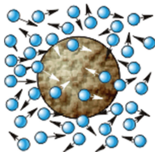
1.2-сурет. Су молекуласының броундық бөлшекпен өзара әсерлесу үлгісі
