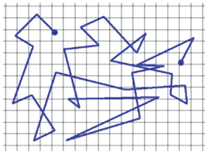
1.1-сурет. Броундық бөлшектердің қозғалыс траекториясы
