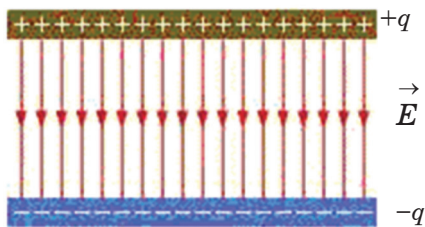
19.6-сурет. Параллель астарлардың арасындағы электр өрісінің кернеулік сызығы
